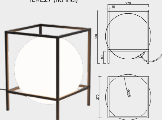
7610 Negro-Black 1LxE27 (no incl)
